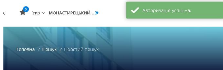
Рис. 3. Успішна авторизація
